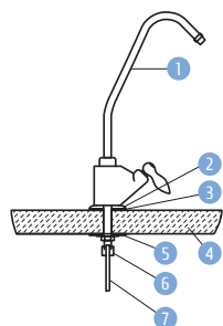
ОДНОЛУЧЕВОЙ КРАН
